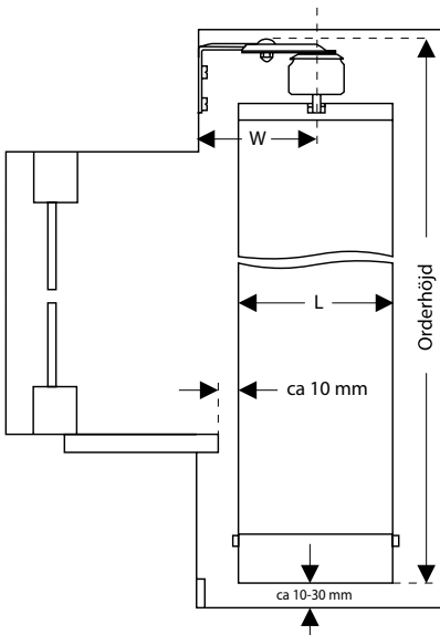
Väggmontage
