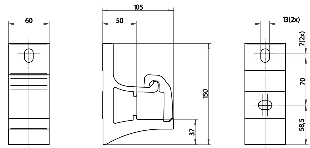
Väggekonsol design
