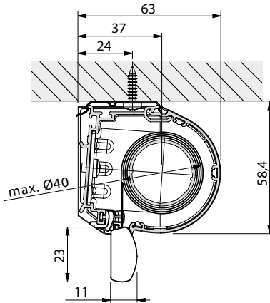
Takmonterad
