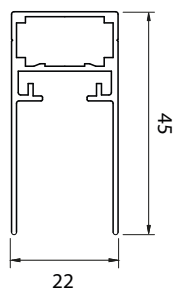
Sido/överlist
