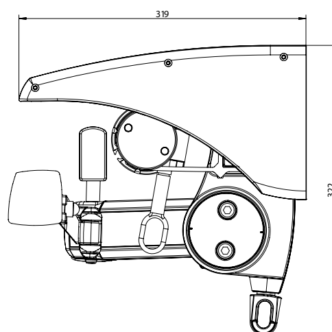
Sidovy T460 Pitcharm inkl. skyddstak
