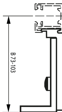
Skenhållare B
