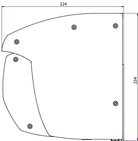
Sidovy T580 vaggmonterad
