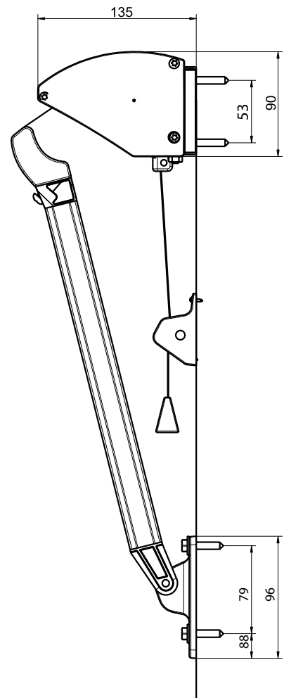
Sidovy F320 inkl. designfront.
