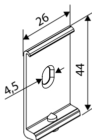
Vevreglage - montageskena
