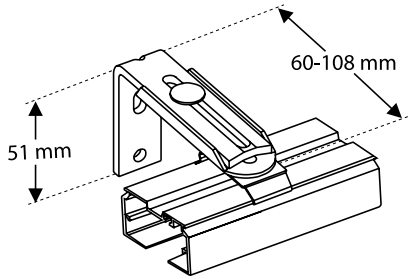
Väggmontage med väggbeslag
