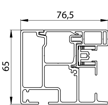
Enkel styrskena
