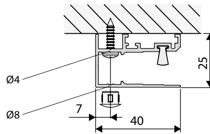
Fördunklande skena Väggmonterad
