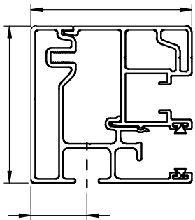
Enkelskena
