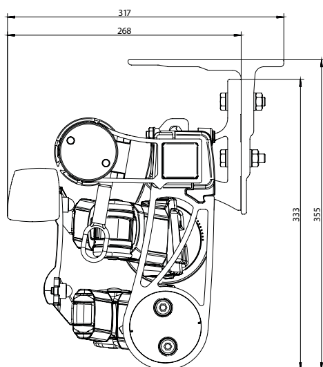
Sidovy T450 + väggkonsol design
