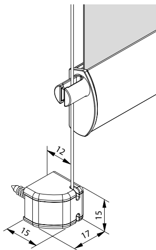
Väggmonterad
