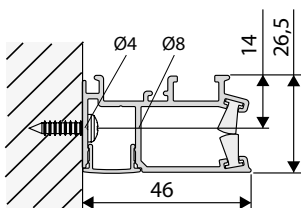
Mörkläggande skena nischmonterad
