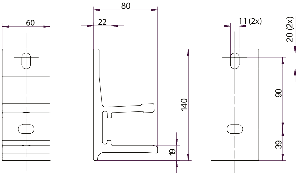
Väggekonsol
