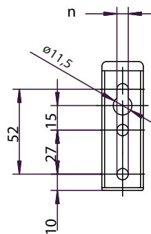
Väggkonsol K10
