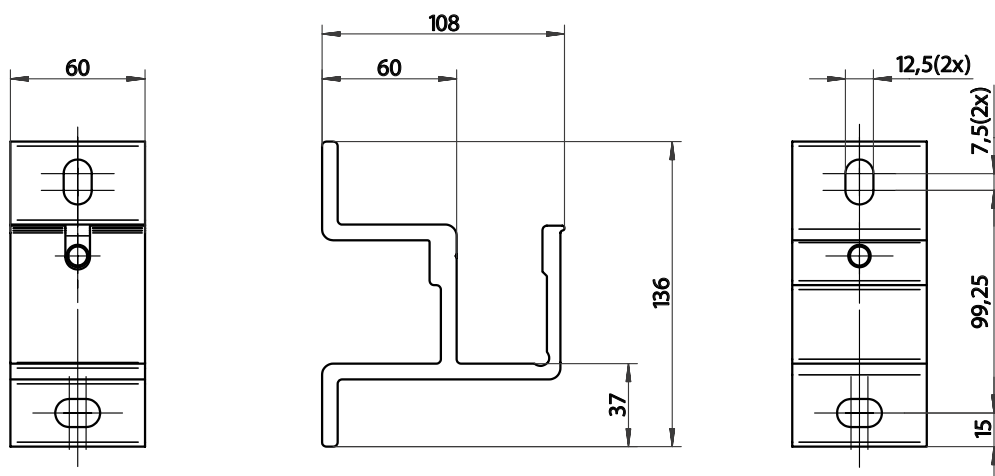
Kombikonsol
