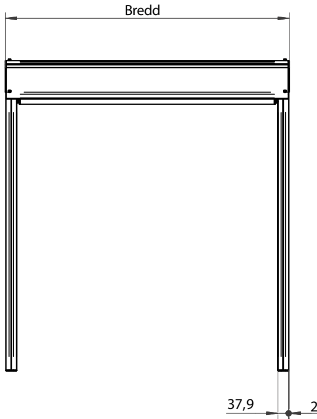
Frontvy S720
