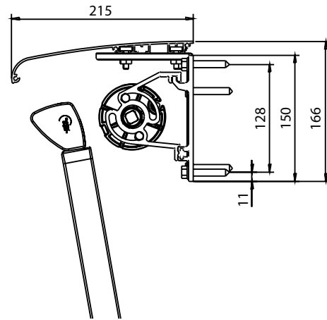
Sidovy F520 inkl skyddstak
