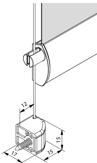
Nischmonterad
