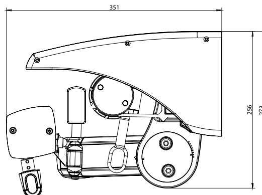
Sidovy T460 Inkl. Skyddstak och rullgardinsfront
