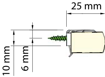
Väggmonterad vid 20/25mm väv
