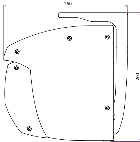
Sidovy T580 takmonterad
