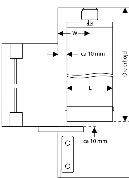
Takmontage mot fönsterbräda
