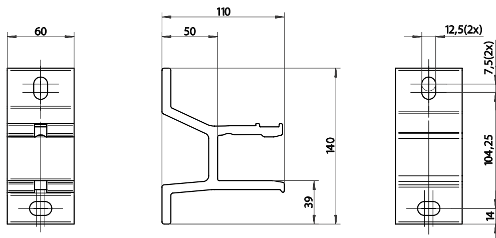
Väggekonsol
