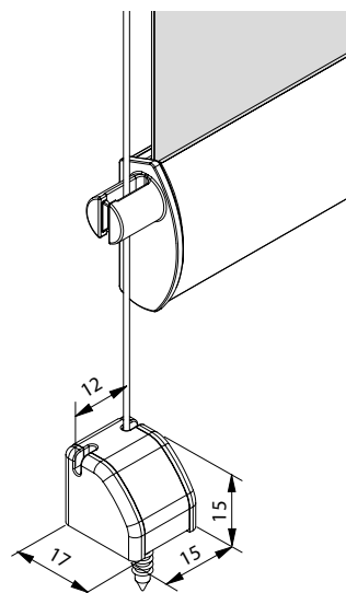
Bottenmonterad
