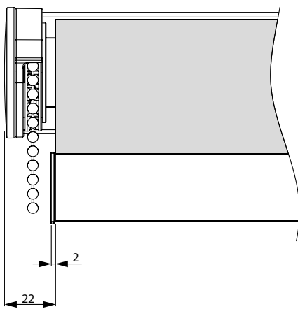
Kulkedja
