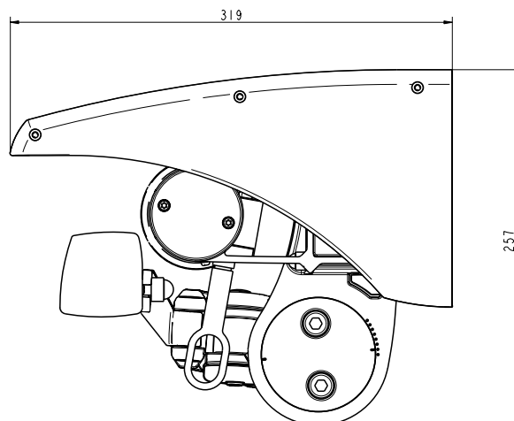
Sidovy T420 Std arm inkl. skyddstak
