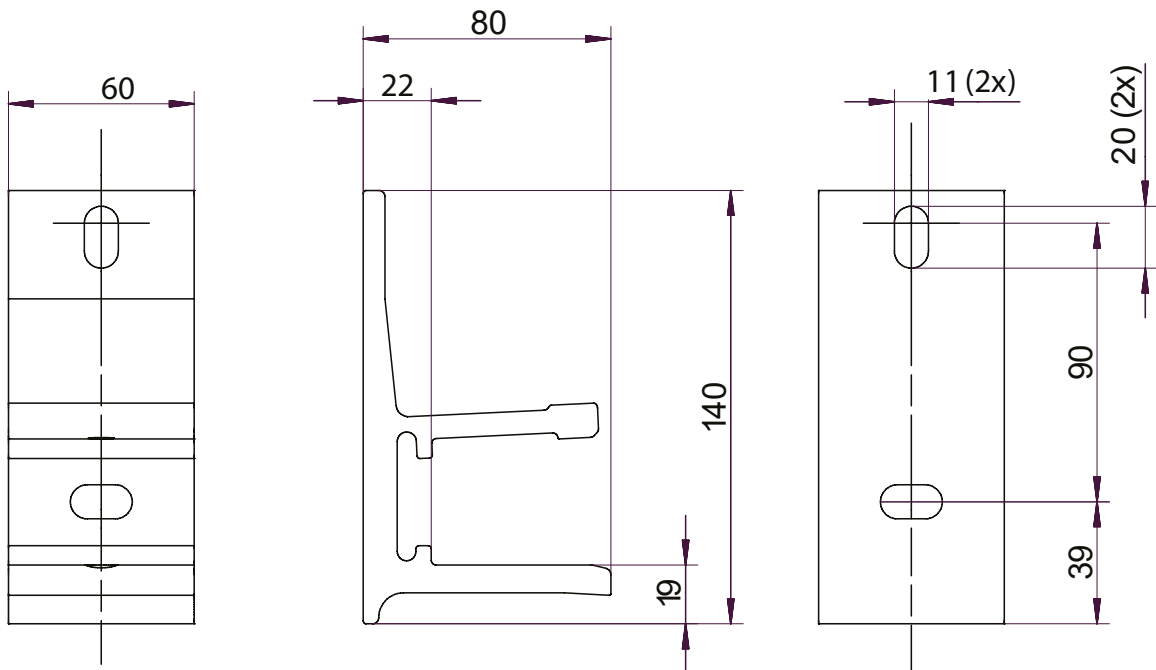
Väggkonsol
