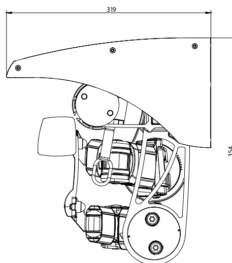
Sidovy T450 inkl. skyddstak
