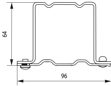
Kassetthållare Tak (standard)
