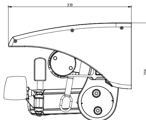
Sidovy T460 Std arm inkl. skyddstak
