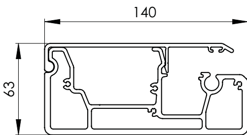
Frontprofil
