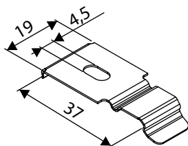
Clips för montageskena
