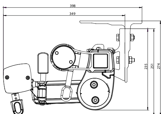
Sidovy T460 Inkl. rullgardinsfront + väggkonsol design
