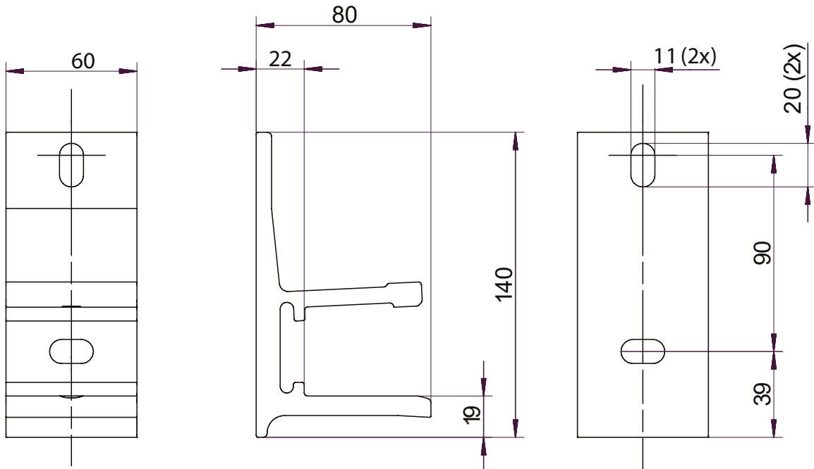
Vaggkonsol
