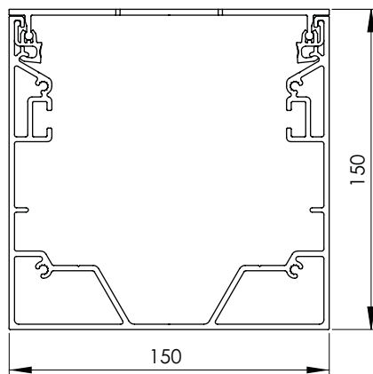
Benprofil
