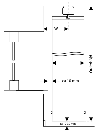
Takmontage
