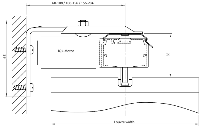
Väggmontage med motor
