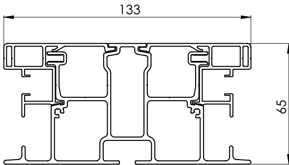
Dubbel styrskena
