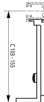
Skenhållare C
