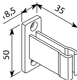
Vevhållare, lång
