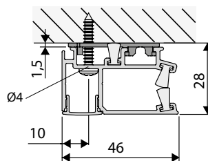
Mörkläggande skena väggmonterad
