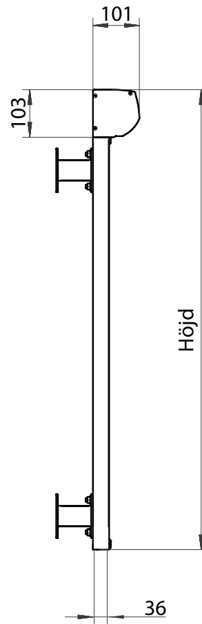
Sidovy S430
