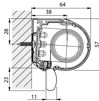
Väggmonterad
