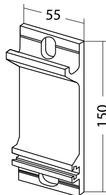
Monteringskonsol Vagg
