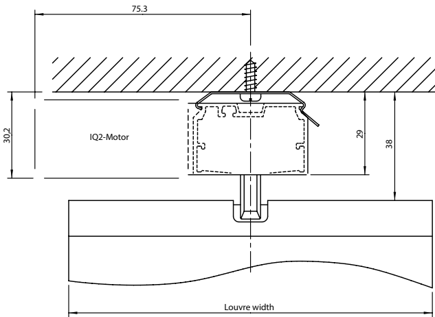
Takmontage med motor
