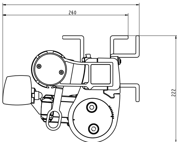
Sidovy T420 Std arm + kombikonsol
