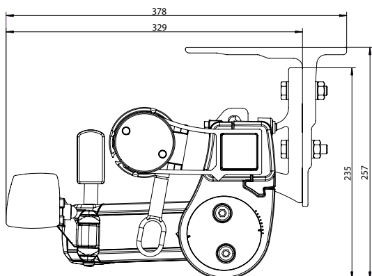
Sidovy T460 Std arm + väggkonsol design
