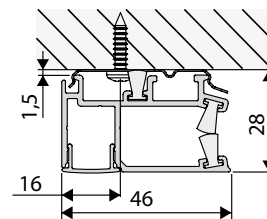
Mörkläggande skena med clips väggmonterad
