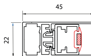
Magnetprofil
