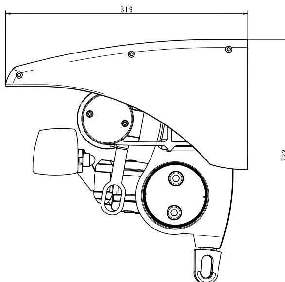
Sidovy T420 Pitcharm inkl. skyddstak
