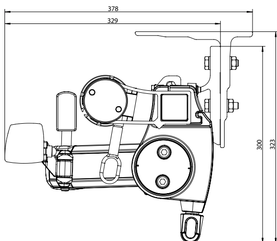
Sidovy T460 Pitcharm + väggkonsol design
