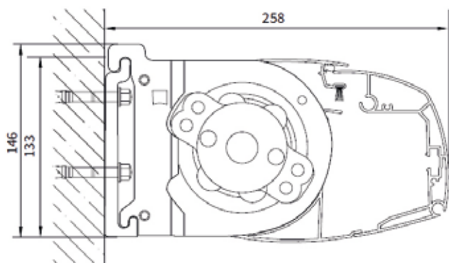
Sidovy T720 + väggkonsol
