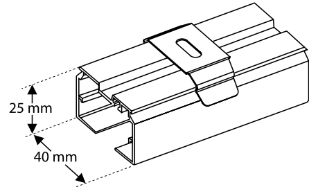
Takmontage med takbeslag
