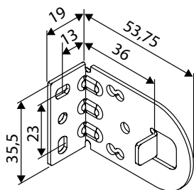
Konsol 36 (standard)
