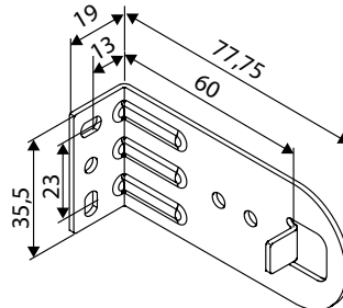
Konsol 60
