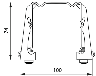
Kassetthållare Tak med snabbfäste
