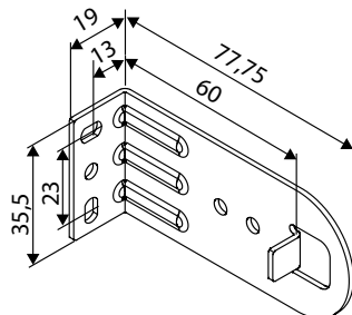
Konsol 60
