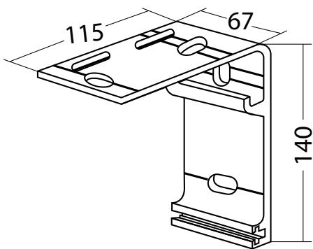
Monteringskonsol Tak
