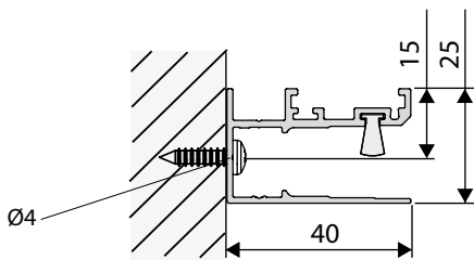
Fördunklande skena Nischmonterad
