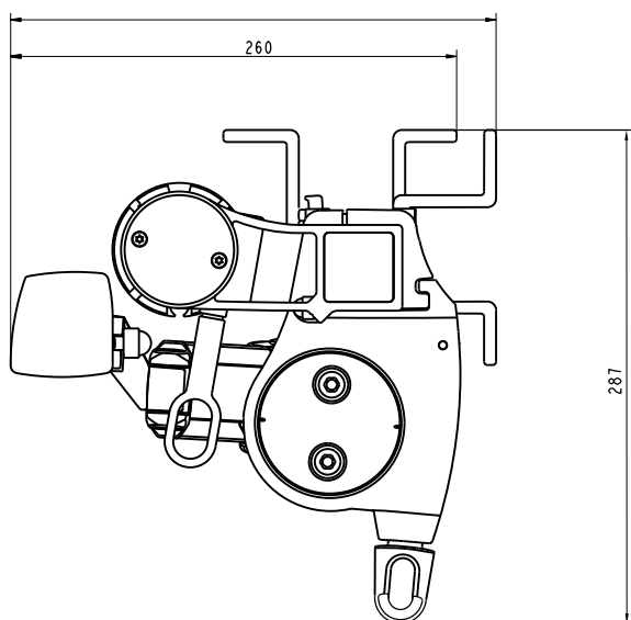
Sidovy T420 Pitcharm + kombikonsol
