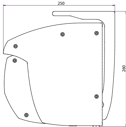
Sidovy T570 takmonterad
