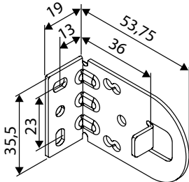
Konsol 36 (standard)
