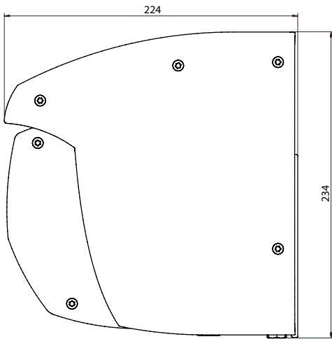
Sidovy T570 väggmonterad
