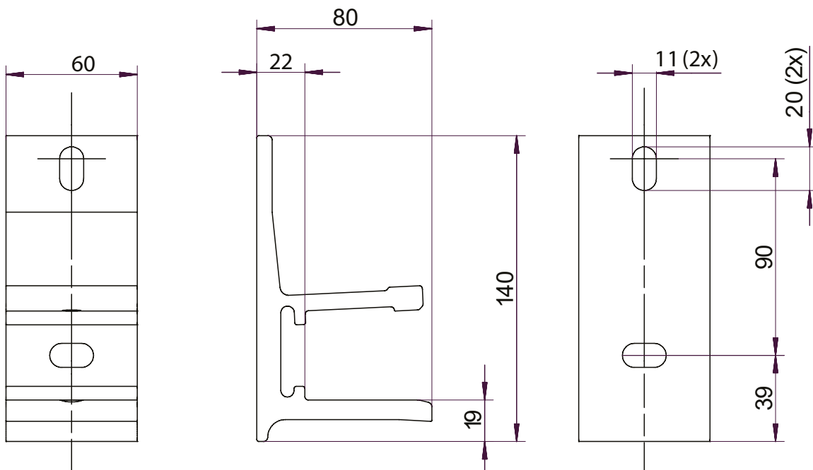
Väggekonsol
