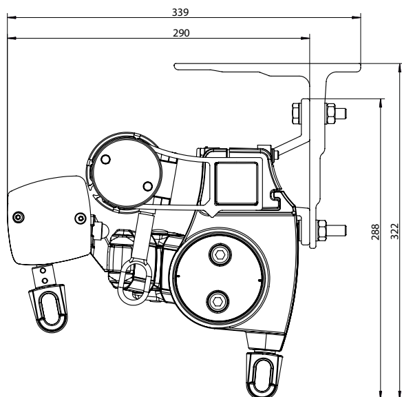
186 Sidovy T420 Pitcharm och rullgardinsfront
